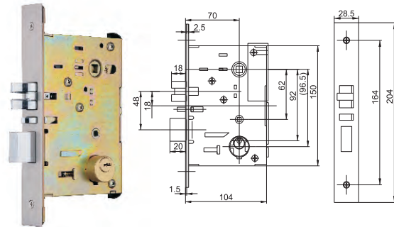
Standard mortise ANSI
